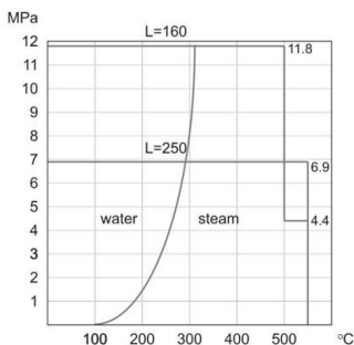
Graph 1. 在 G1 和 T1 屏蔽工作条件下允许的负载 - 15 HM, 1H18N9T, H17N13M2T
