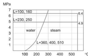
Graph 2. 在 GN1 和 GB1 屏蔽工作条件下允许的负载 - 15 HM 1H18N9T H17N13M2T
